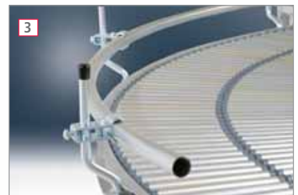
3 Seitenführungen aus Stahlrohr 25 mm Ø verzinkt. Stufenlos höhenverstellbar von 50–130 mm. Breite stufenlos verstellbar von Bahn-Nutbreite -140 bis +24 mm.
